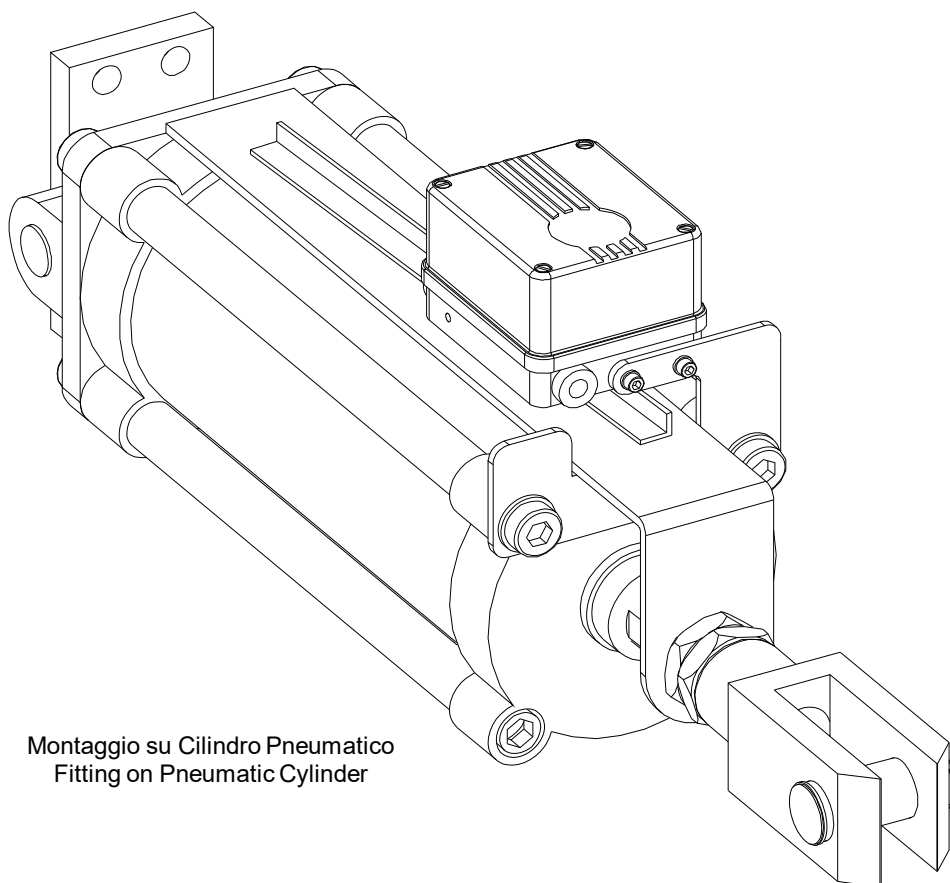
Fixing kit 072-55 Kit di fissaggio 072-55
