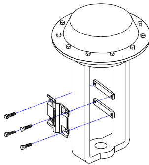
Fixing kit 973SUP Kit di fissaggio 973SUP
