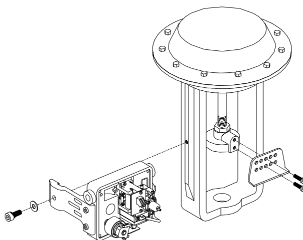
Standard Fixing kit Kit di fissaggio standard
