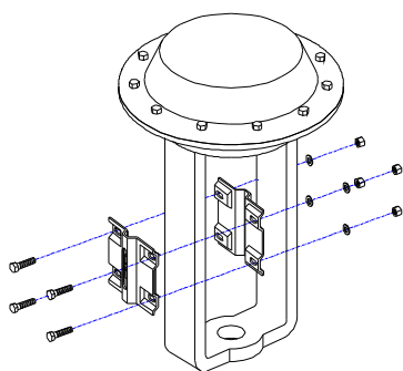
Fixing kit 072-55 Kit di fissaggio 072-55
