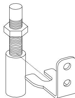
Valve spindle adaptor 180-23 Adattatore perno di feedback 180-23
